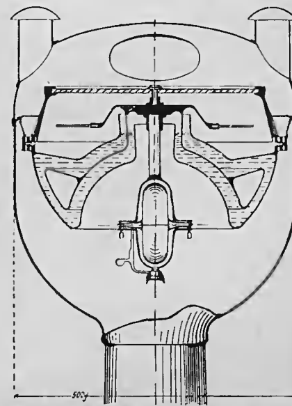
3. Общая схема укрѣпленія частей въ компасѣ Аншютца.
